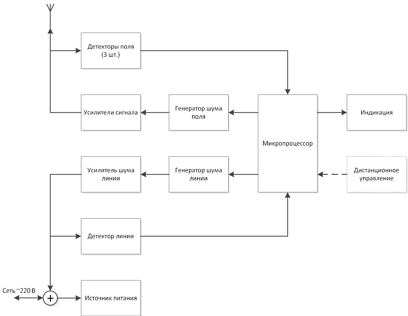
Рисунок 1 – Функциональная схема
